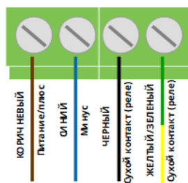
КЛЕММНИК НА СМАРТ ПРИЕМНИКЕ
